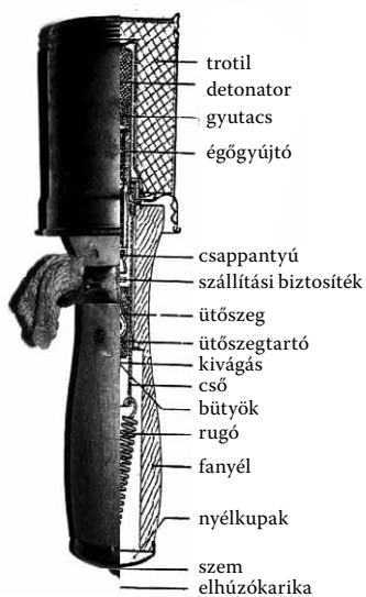
13. ábra. A kézigránát általános felépítése
